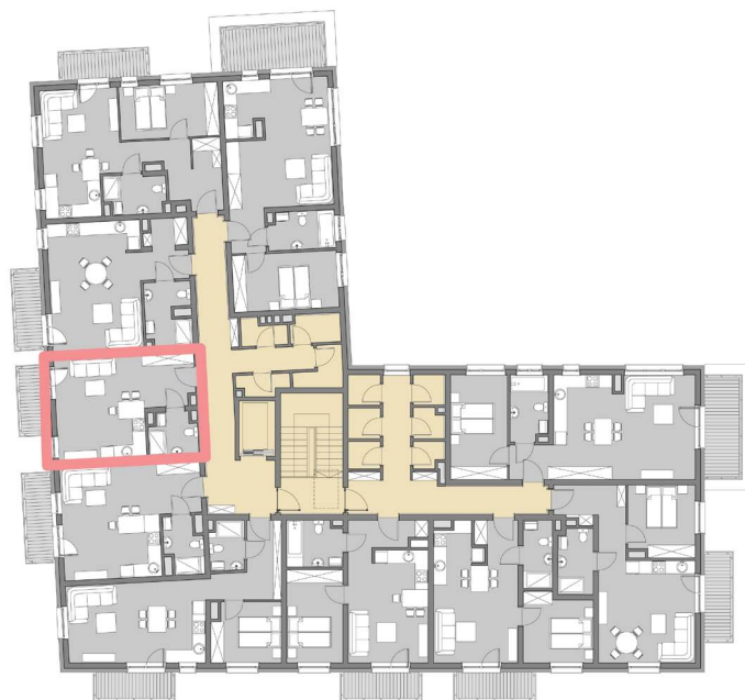
RZUT KONDYGNACJI: PIĘTRO III
