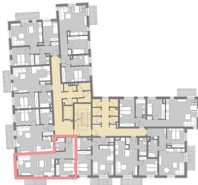
RZUT KONDYGNACJI: PIĘTRO II
