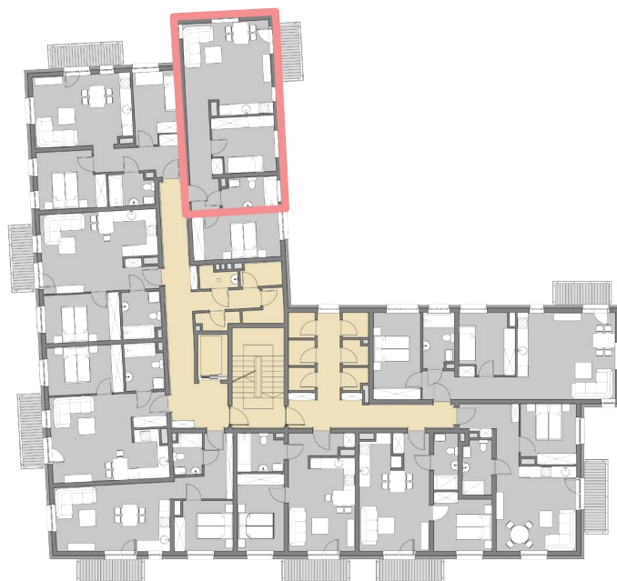
RZUT KONDYGNACJI: PIĘTRO I
